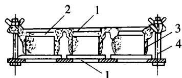
图 T 0145-12 并列式饱和器
