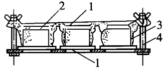
图 T 0146-12 平行式饱和器 1-夹板;2-透水石;3-环刀;4-拉杆
