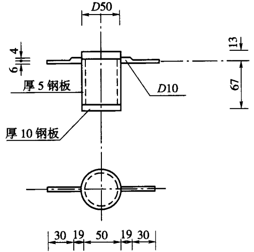
图 T 0136-2 承载板(单位:mm)
