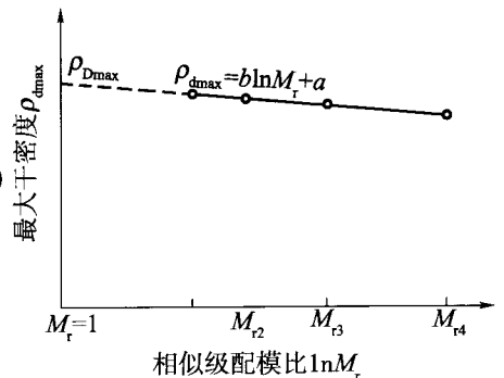
图 T 0132-3 模型料 \rho_{\text{dmax}} - M_r 关系
