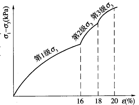
图 T 0177-8 按轴向应变加荷
