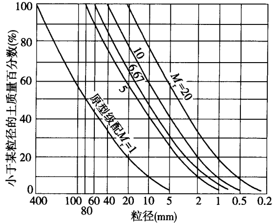
图 T 0133-2 原型料与模型料级配关系
