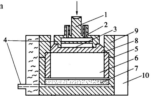
图 T 0188-1 融化压缩仪示意图
