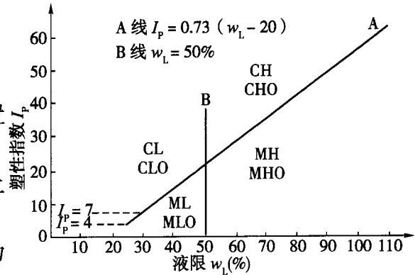
图 3-7 塑性图
