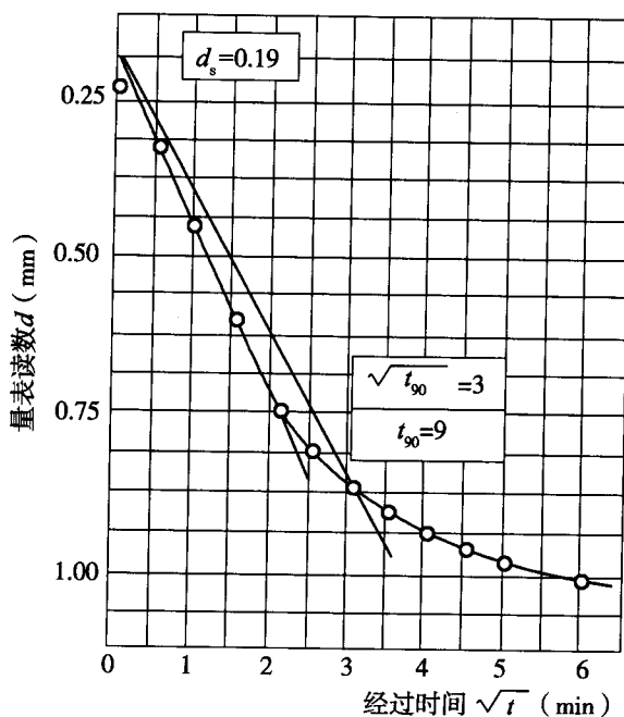
图 T 0138-3 用时间平方根法求 t_{90}
