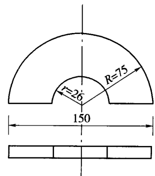
图 T 0134-5 荷载板(单位:mm)
