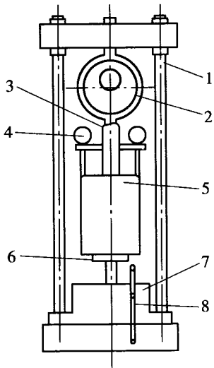
图 T 0134-2 手摇测力计式载荷装置示意图
