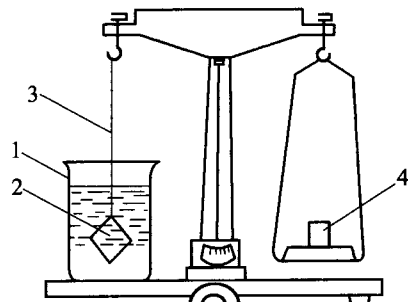
图 T 0179-1 浮重天平
