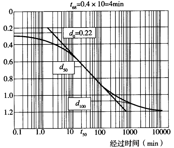
图 T 0137-4 用时间对数坡度法求 t_{68}
