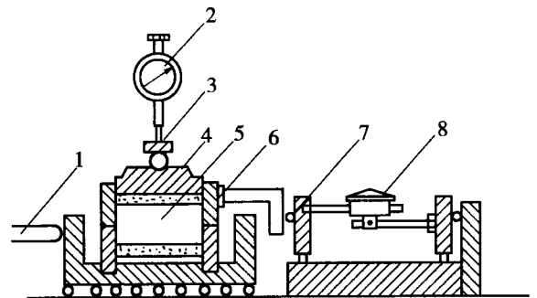
图 T 0142-1 应变控制式直剪仪示意图
