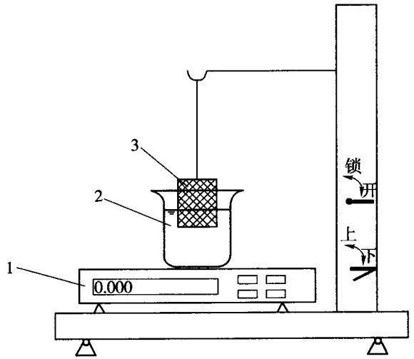
图 T 0169-1 浮力仪
