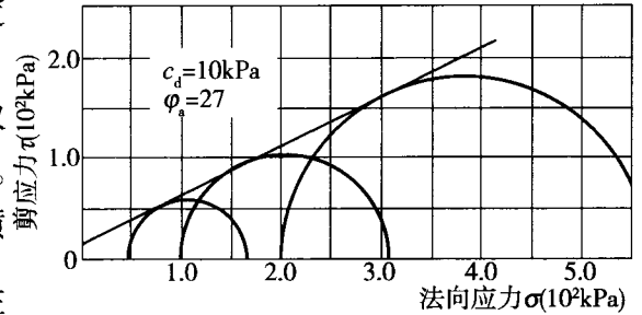
图 T 0146-13 固结水排强度包线
