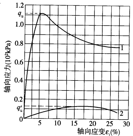
图 T 0148-4 轴向应力与应变的关系曲线 1-原状试样；2-重塑试样
