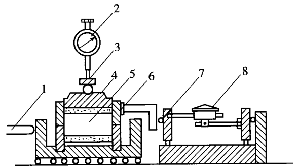
图 T 0143-1 应变控制式直剪仪示意图
