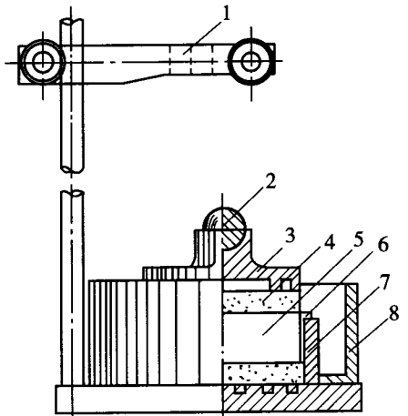
图 T 0137-1 固结仪
