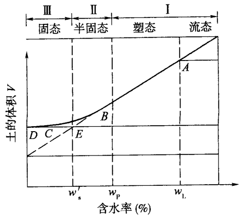
图 T 0121-3 土体收缩过程
