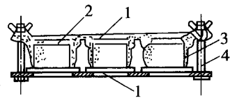
图 T 0177-4 平列式饱和器
