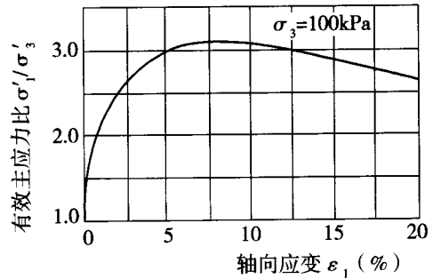
图 T 0145-14 有效主应力比与轴向应变的关系曲线
