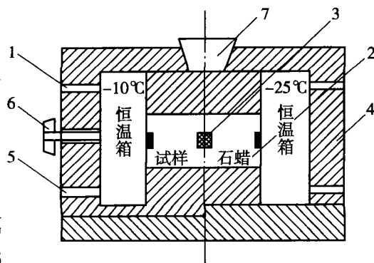
图 T 0185-1 导热系数试验装置示意图 1-冷浴循环液出口;2-试样盒;3-热电偶;4-保温材料;5-冷浴循环液进口;6-夹紧螺杆;7-保温盖
