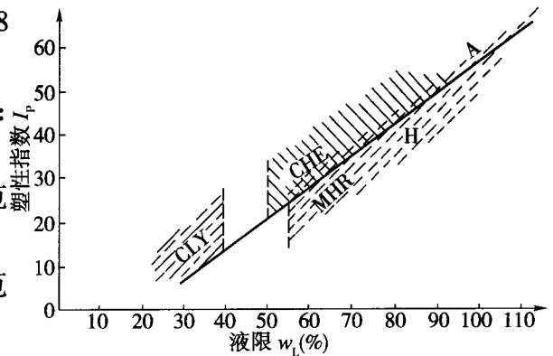
图 3-8 特殊土塑性图
