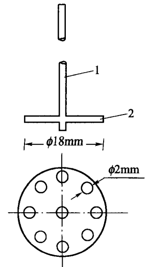
图 T 0124-1 搅拌器示意图 1-直杆;2-圆盘
