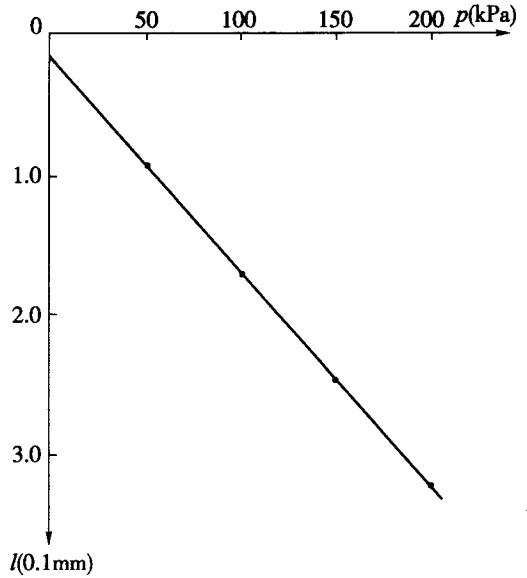
图 T 0135-3 单位压力与回弹变形( p-l )的关系曲线
