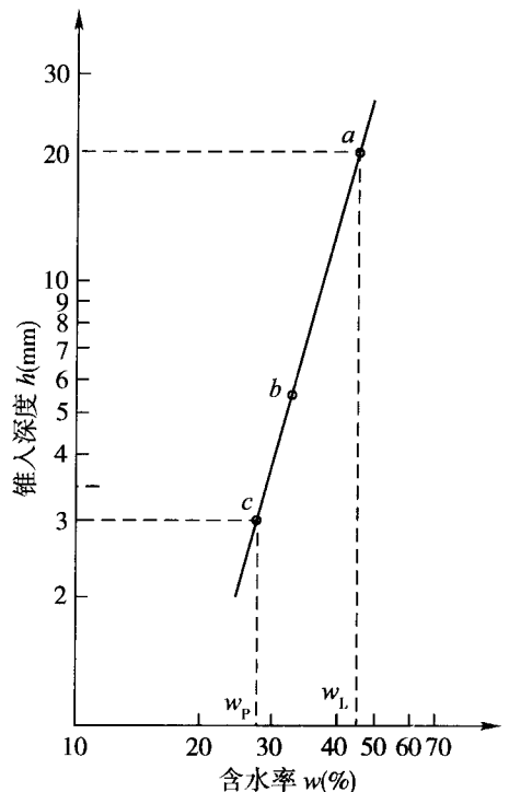
图 T 0118-1 锥入深度与含水率( h-w )关系
