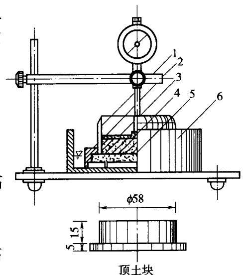
图 T 0126-1 膨胀仪(单位:mm)
