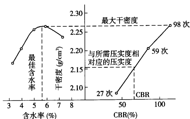
图 T 0134-7 对应于所需压实度的 CBR 求取方法
