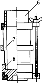
图 T 0145-2 击实器
