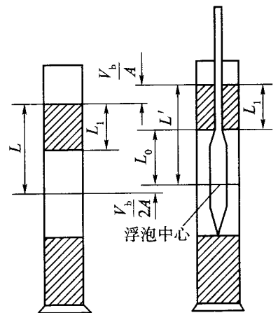
图 T 0116-4 土粒有效沉降距离校正
