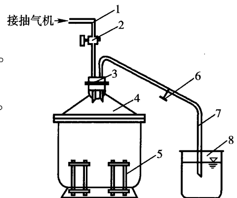
图 T 0102-4 真空饱和法装置
