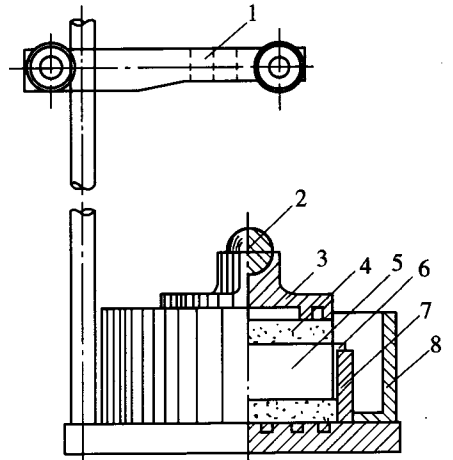
图 T 0139-1 固结仪
