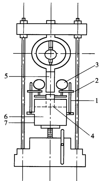
图 T 0136-1 路面材料强度仪 及试样安装方法
