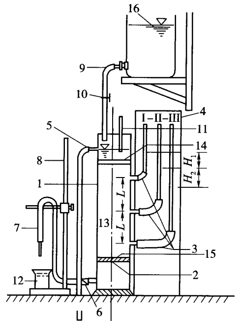
图 T 0129-1 常水头渗透仪装置
