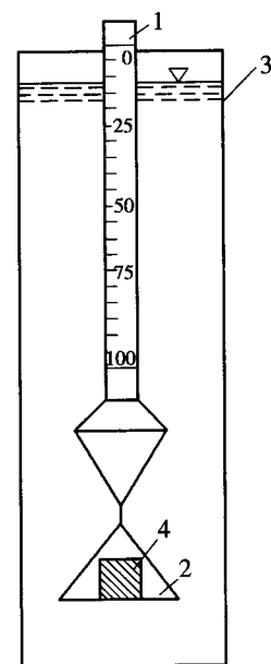
图 T 0171-1 湿化仪示意图
