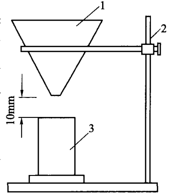
图 T 0124-2 量样装置 1-漏斗;2-支架;3-量土杯
