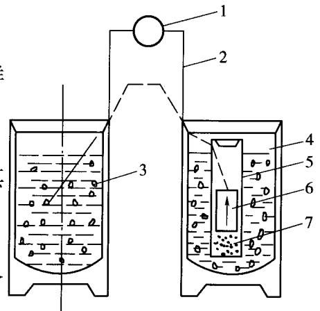
图 T 0184-1 冻结温度试验装置示意图
