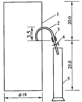
图 T 0114-1 虹吸筒(单位:cm)
