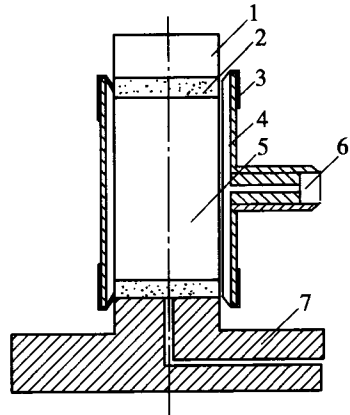
图 T 0144-7 承膜筒
