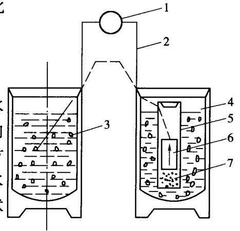
图 T 0186-1 冻结温度试验装置示意图
