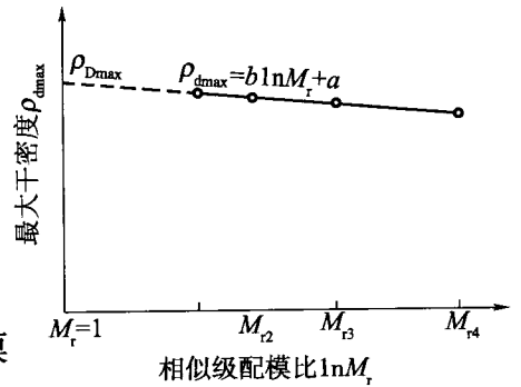
图 T 0133-3 模型料 \rho_{dmax} - M_r 关系
