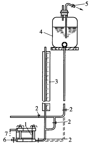
图 T 0130-2 变水头渗透装置
