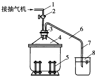
图 T 0177-1 真空饱和法装置
