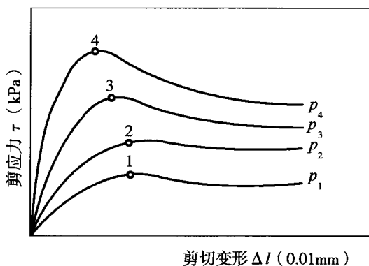
图 T 0141-2 剪应力 \tau 与剪切位移 \Delta l 的关系曲线
