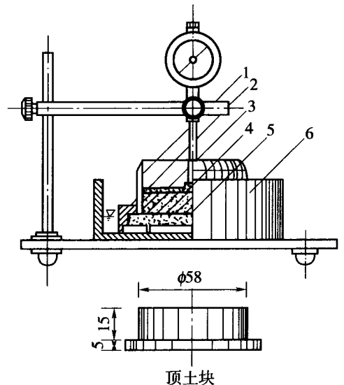
图 T 0125-1 膨胀仪(单位:mm)
