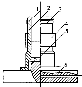
图 T 0145-8 对开圆模
