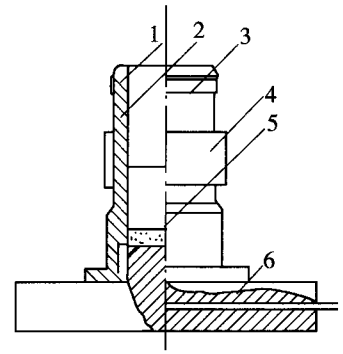
图 T0144-8 对开圆膜
