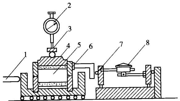
图 T 0141-1 应变控制式直剪仪示意图
