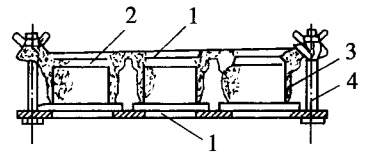
图 T 0144-12 并列式饱和器
