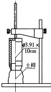
图 T 0146-5 切土器
