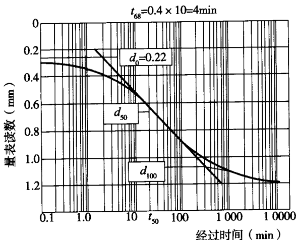
图 T 0138-4 用时间对数坡度法求 t_{68}
