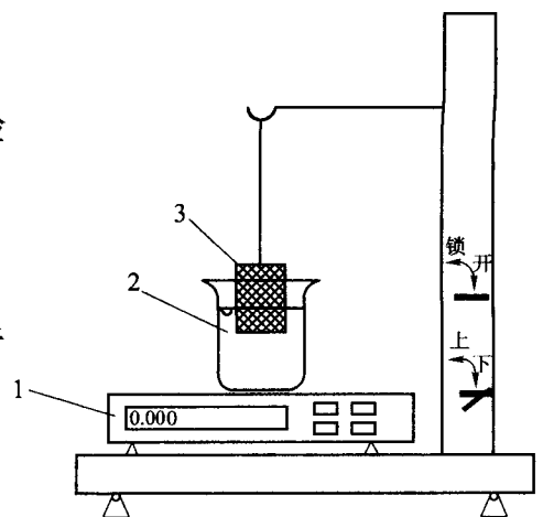
图 T 0180-1 浮力仪
