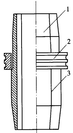
图 T 0148-3 重塑筒 1-重塑筒筒身(可以拆成两半);2-钢箍;3-接缝
