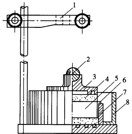
图 T 0138-1 固结仪
